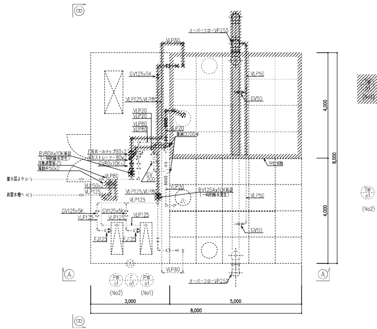
平面図 1: 50 注) 受水槽No1撤去にあたり水櫃内水抜き・中仕切板補強を行うこと。 配管撤去にあたりアスベスト除去・処分を行うこと。
