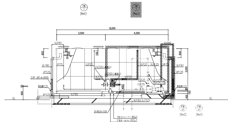
⑧—⑧ 断面图 1:50
