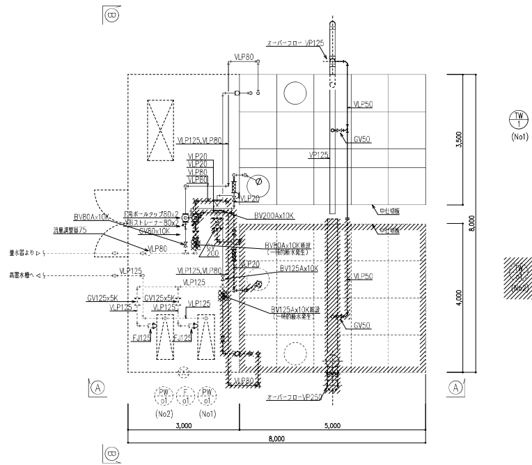
平面図 1 : 50
