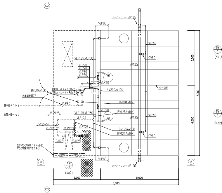
平面図 1 : 50
