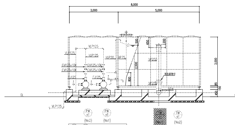
①—① 断面图 1:50
