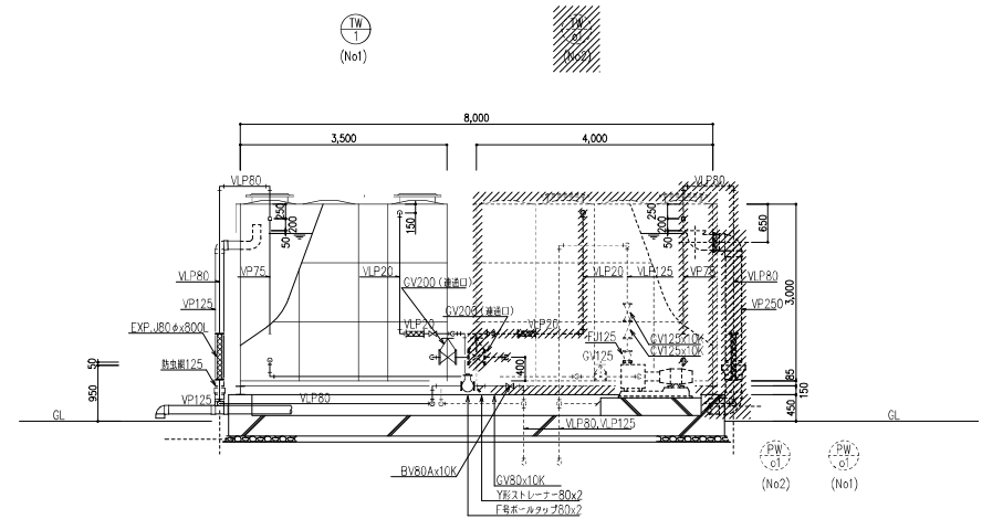
(B) - (B) 断面図 1 : 50
