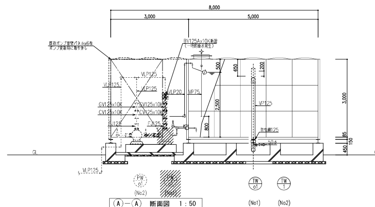
①—① 断面图 1:50
