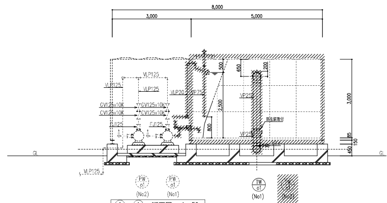
(A) - (A) 断面図 1 : 50
