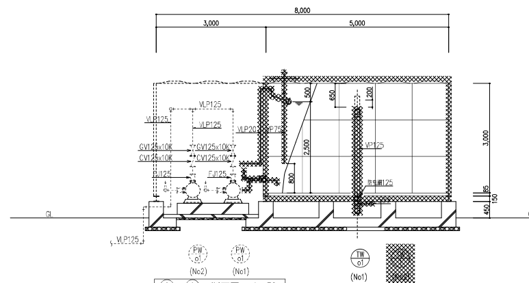
①—① 断面图 1:50
